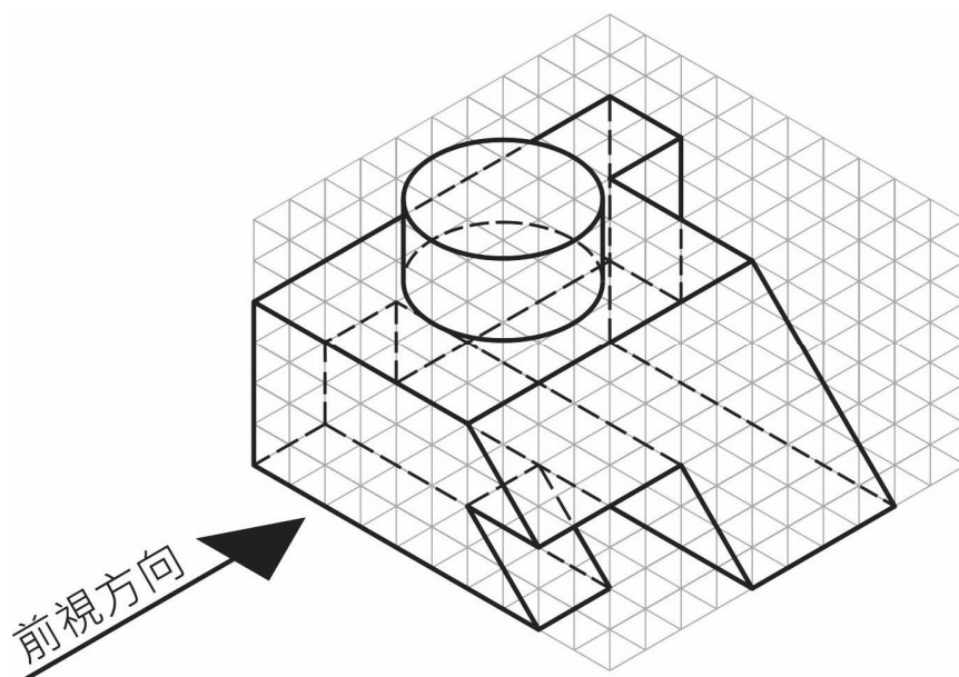
圖(一) 等角立體圖，圖底的參考格線每格為 5 mm
