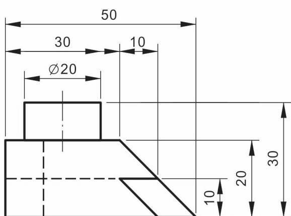
前視圖
